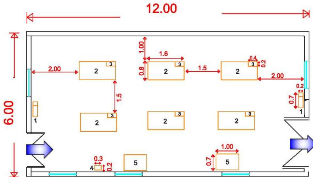
چیدمان تجهیزات کارگاه حرفه آزمایشگر قطعات صنعتی با مایع نافذ (PT)
